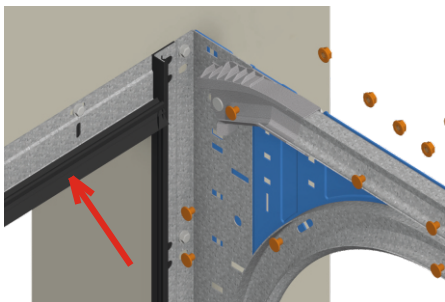
Překladový profil s horním těsněním
