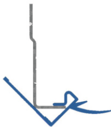
Detail uchycení těsnění
